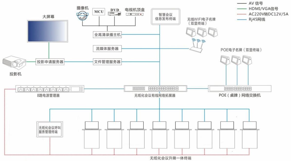
智能无纸化会议系统原理图
