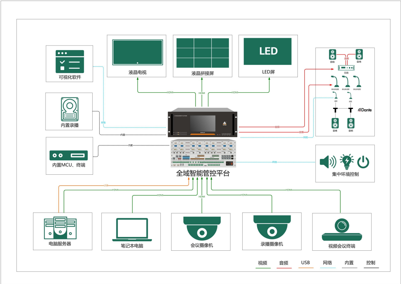
多媒体会议系统拓扑图
